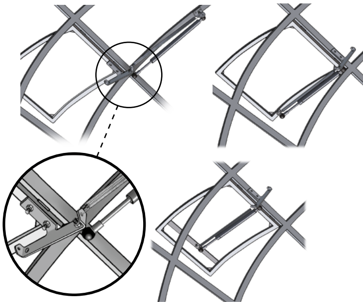
Установка на подъёмную (вертикальную) форточку
